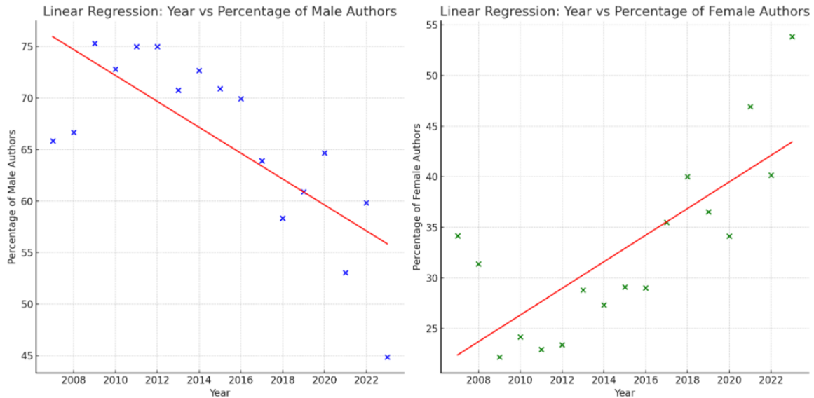
Figuur 5: overzicht correlatietoets gemiddeld percentage recensies over boeken van mannelijke en vrouwelijke auteurs in de periode 2007-2023
