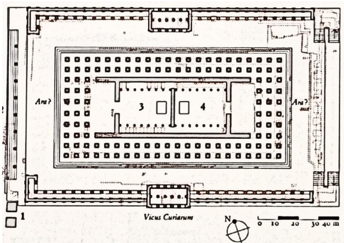
Afb. 9a: Reconstructie van het grondplan van de Tempel van Venus en Rome in zijn Hadrianische fase (Tekening: F. Fraioli, La città e le sue parti: Regione IV, Templum Pacis , in: A. Carandini en P. Carafa red., Atlante di Roma antica: Biografia e ritratti della città. 1: Testi e immagini (Milaan 2012) 102.
