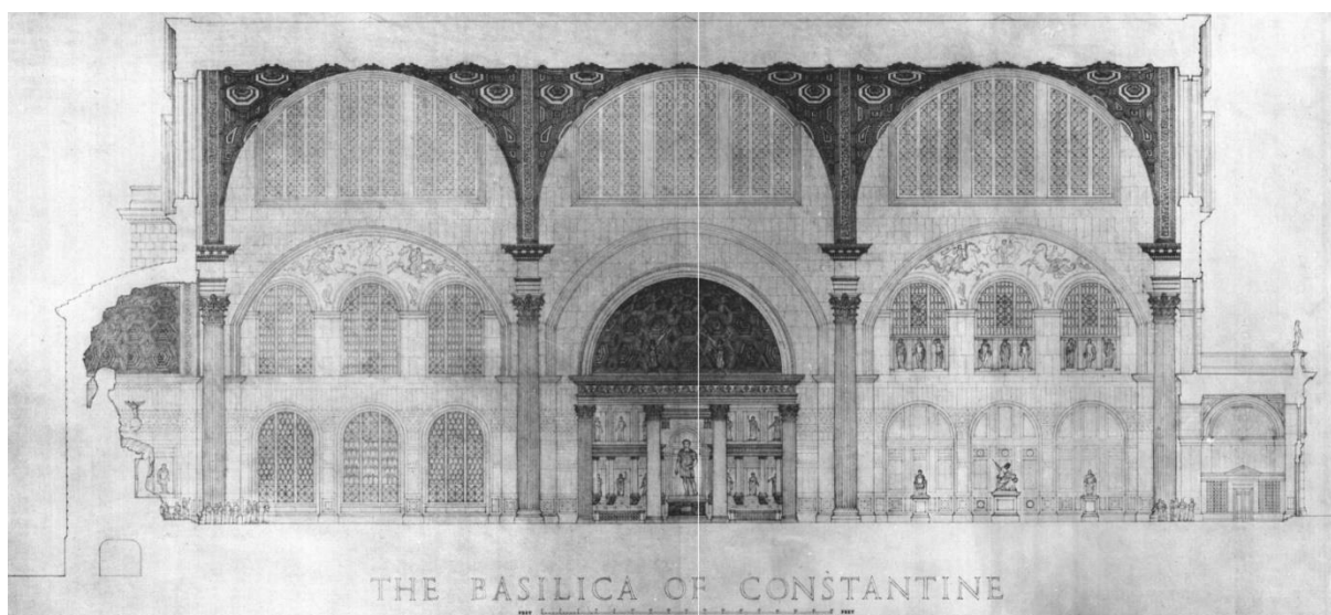
Afb. 4: Reconstructie binnenzijde van de Basilica Nova gezien vanaf de zuidzijde naar de door Constantijn aangebouwde apsis. Aan de linkerkant is de locatie van een enorm standbeeld aangegeven van Maxentius/Constantijn (Tekening van Anthony Minoprio, 'A Restoration of the Basilica of Constantine, Rome', Papers of the British School at Rome Vol.12 (1932) 51-52.
