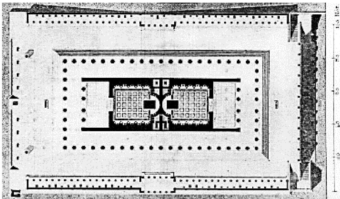
Afb. 9b: Reconstructie van het grondplan van de Tempel van Venus en Roma in zijn Maxentische fase (Tekening Léon Vaudoyer 1830)
