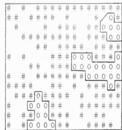
Figuur 1.1.1 Equilibrium vanuit een willekeurige verdeling met een minderheid die veeleisender is dan de meerderheid (Schelling, 1971)
