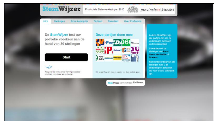
Afbeelding 1. Schermweergave 'Intro'
