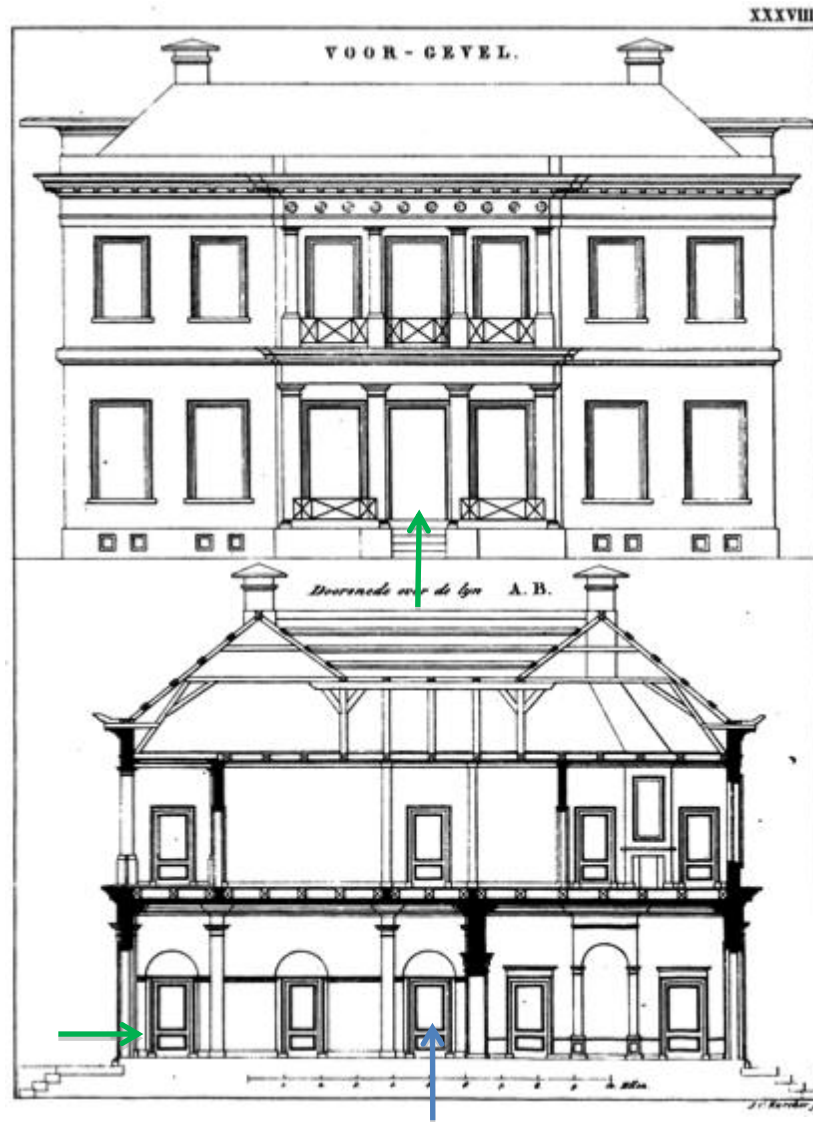
Afbeelding 81, 82 en 83: prent XXXVIII, XXXVII, XXXVI; gevel, doorsnede, plattegrond begane grond. Plattegrond verdieping.
