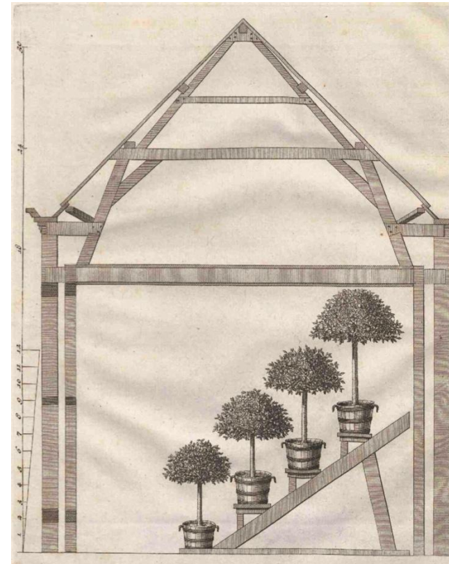
Afbeelding 15, voorbeeld van een oranjerie.
