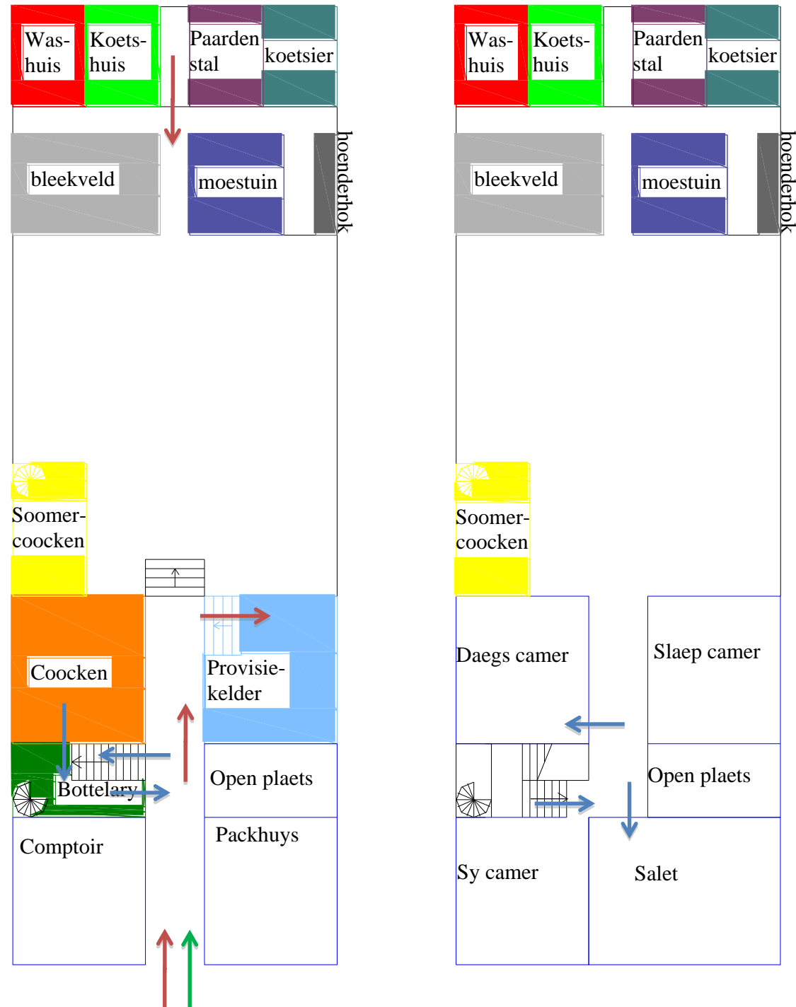
Ideale situatie zeventiende-eeuws stadshuis type begane grond – eerste verdieping
