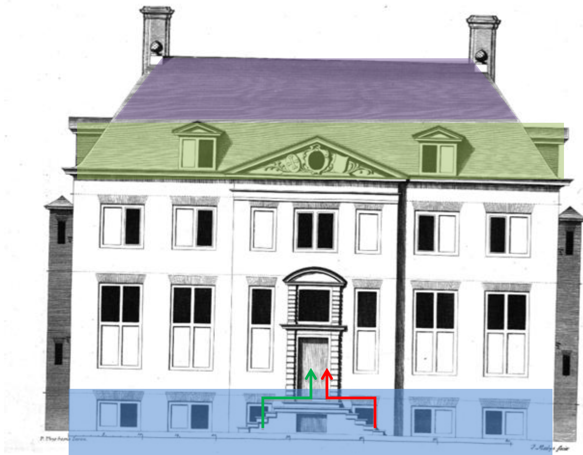
Afbeelding 21: Prent 6; Voorgevel.
