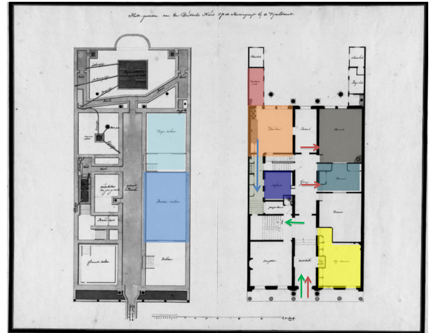
Afbeelding 68: plattegrond riolering met kelders en begane grond door Van der Hart (1791).
