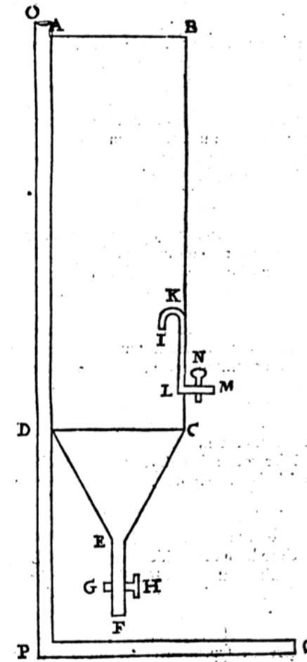
Afbeelding 13: doorsnede pompkraan en methode om slijk weg te spoelen.
