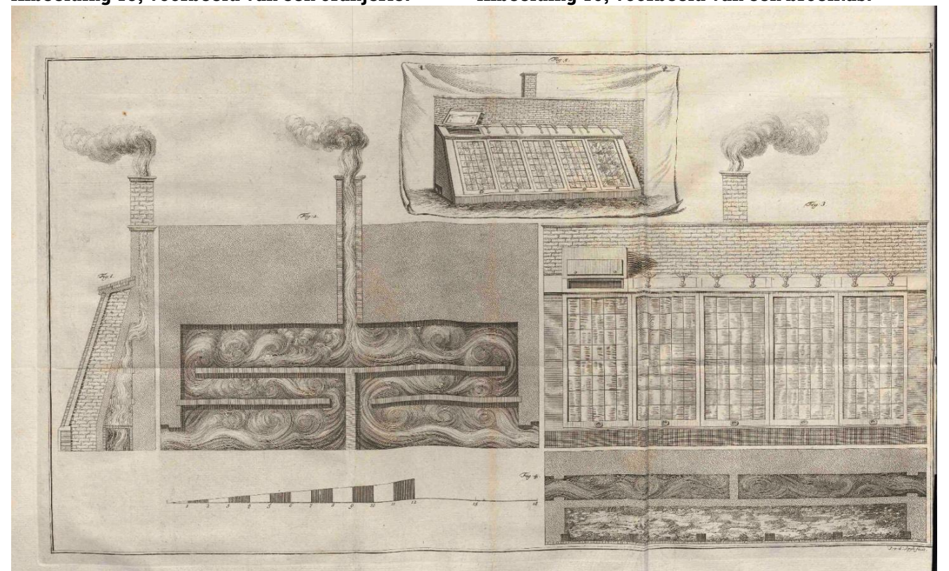
Afbeelding 17, voorbeeld van een broeikas.
