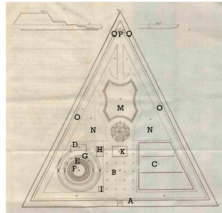
Afbeelding 11: De ideale schikking volgens De la Court.
