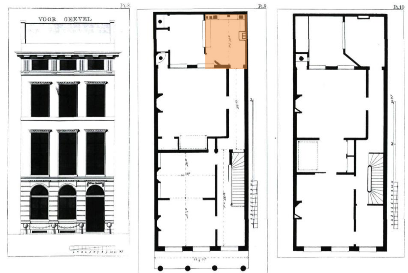
Afbeelding 61, 62 en 63: opstand en plattegrond begane grond en verdieping vierde huis van Van Straaten.
