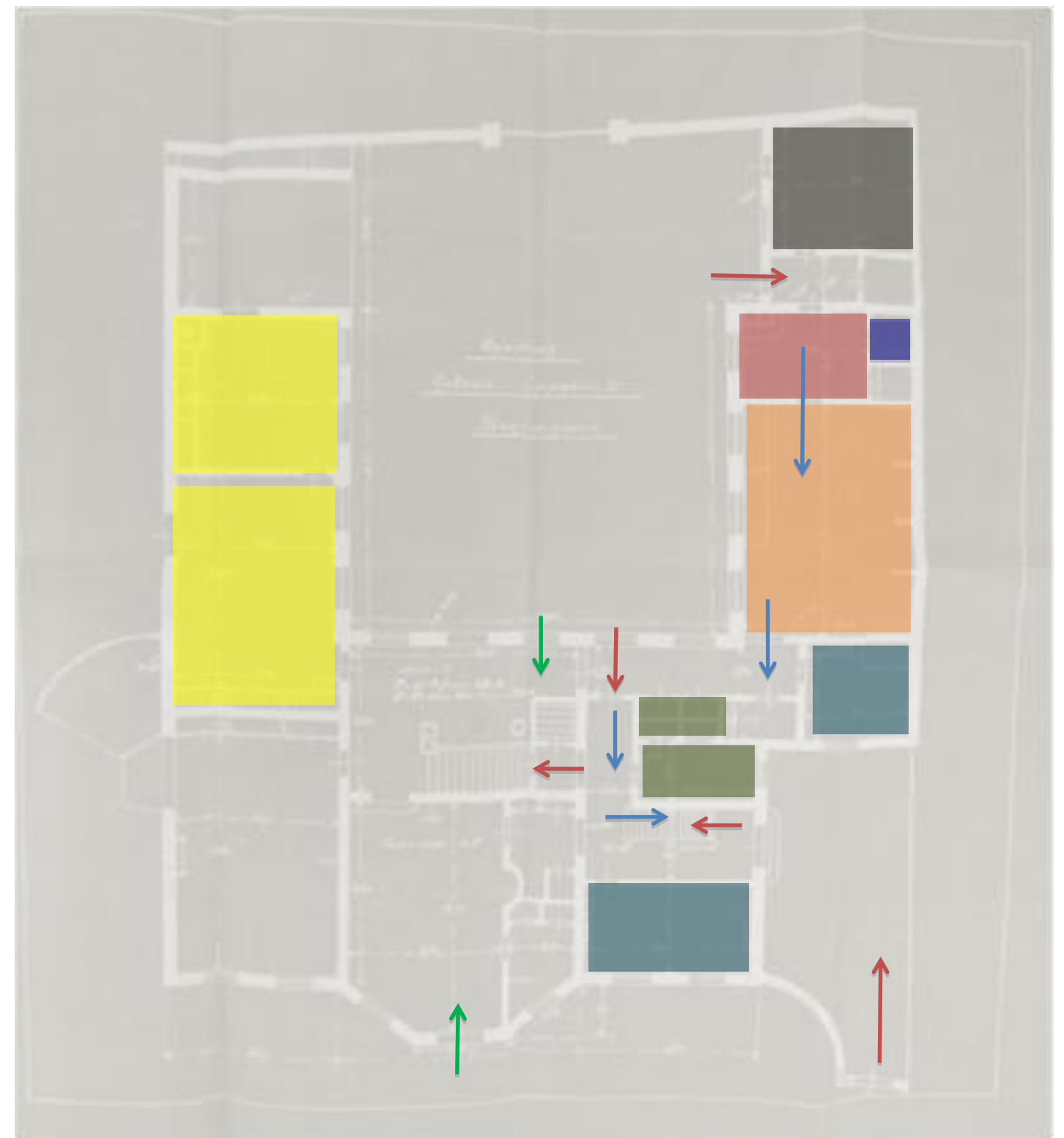
Afbeelding 71 en 72: plattegrond riolering met kelders en begane grond door Van der Hart (1794).
