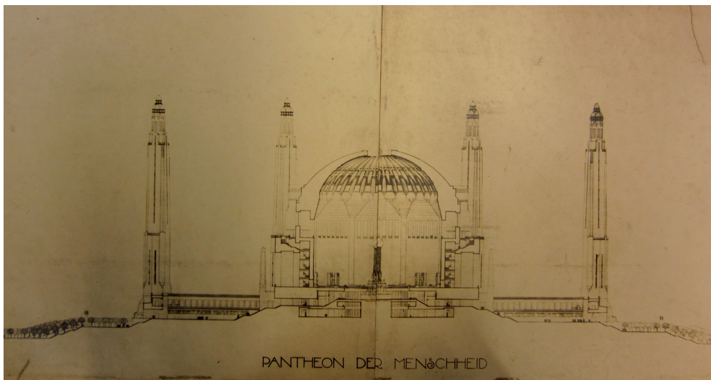
Afbeelding 10. Tekening doorsnede tempel 1915 van H.P. Berlage, Bron: Nederlands Architectuur Instituut, Rotterdam, Archief BERL 154. Foto: auteur.
