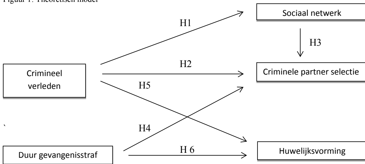
Figuur 1: Theoretisch model
